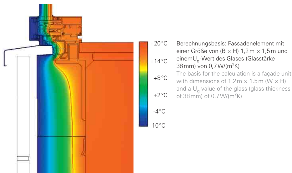
Isothermverlauf der Schüco FWS 60 CV.HI Fassade bei einem U_{cw} -Wert von 0,84 \text{ W}/(\text{m}^2\text{K}) Isothermal flow of the Schüco FWS 60 CV.HI façade with a U_{cw} value of 0,84 \text{ W}/(\text{m}^2\text{K})
