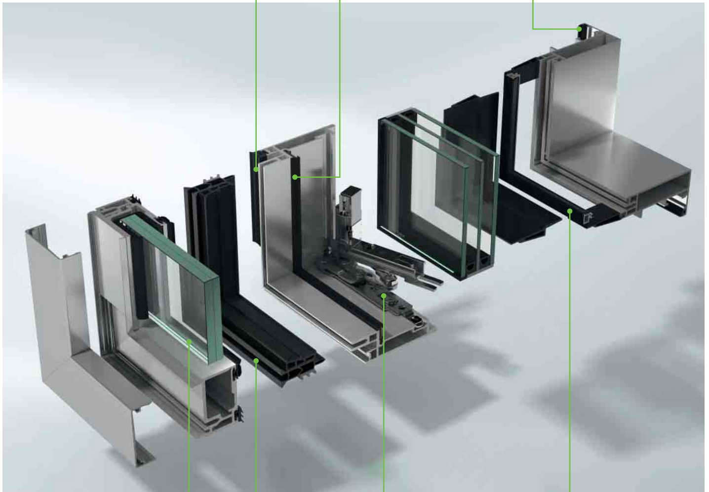
Profilintegrierte Brüstungsverglasung Spandrel glazing integrated in the profile
