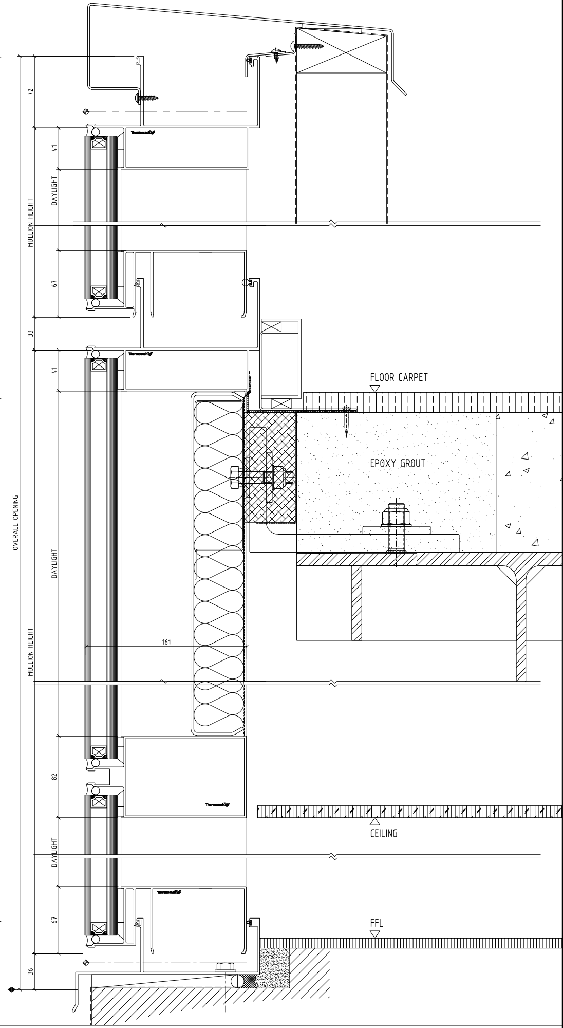
04 HEAD 1:2
