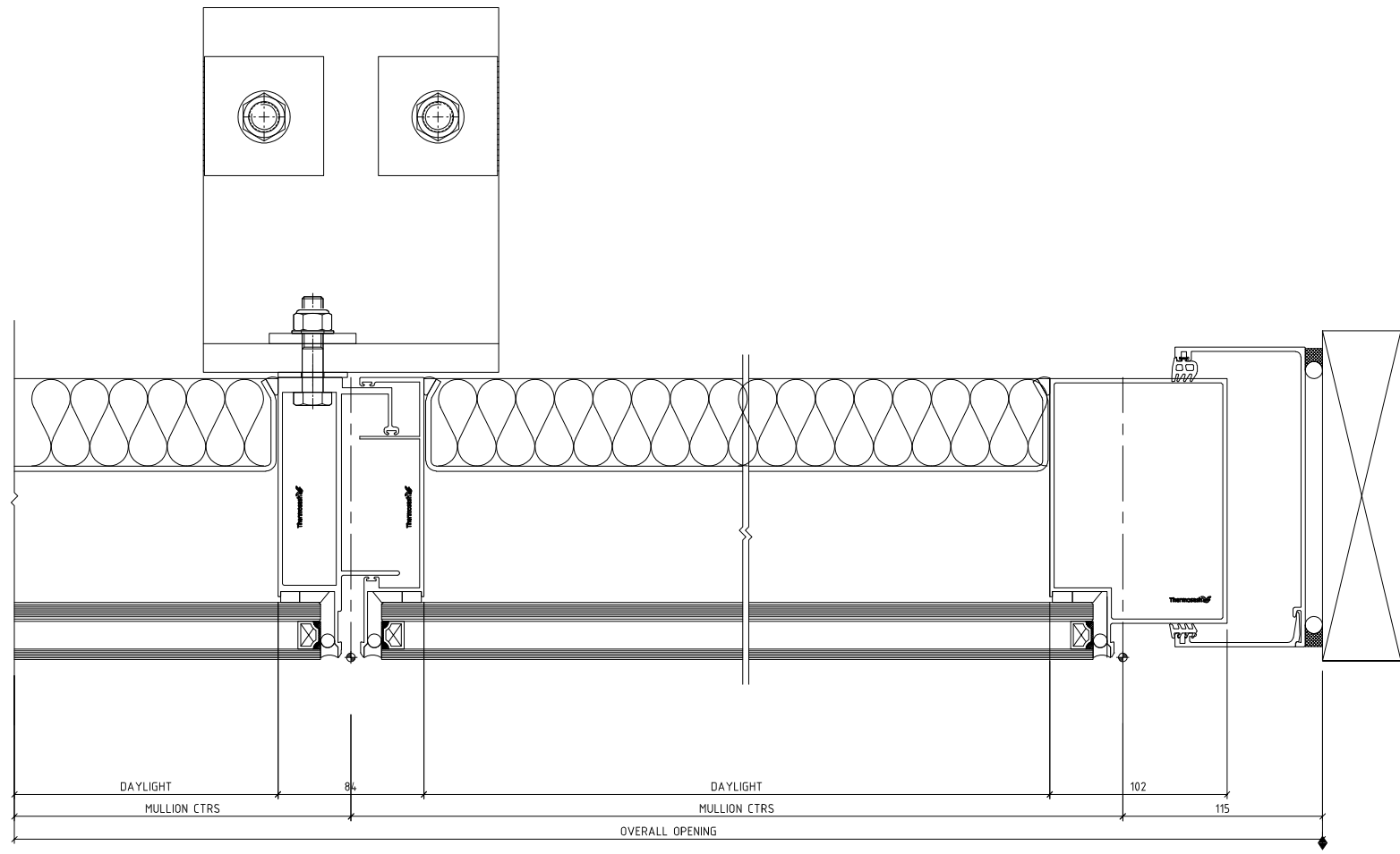
05 MULLION 1:2 06 JAMB 1:2
