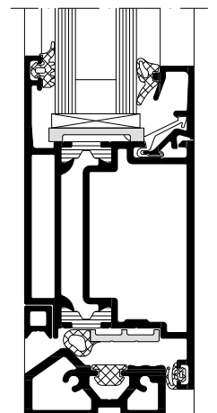
Schüco Tür ADS 50, Maßstab 1:2 Schüco Door ADS 50, scale 1:2
