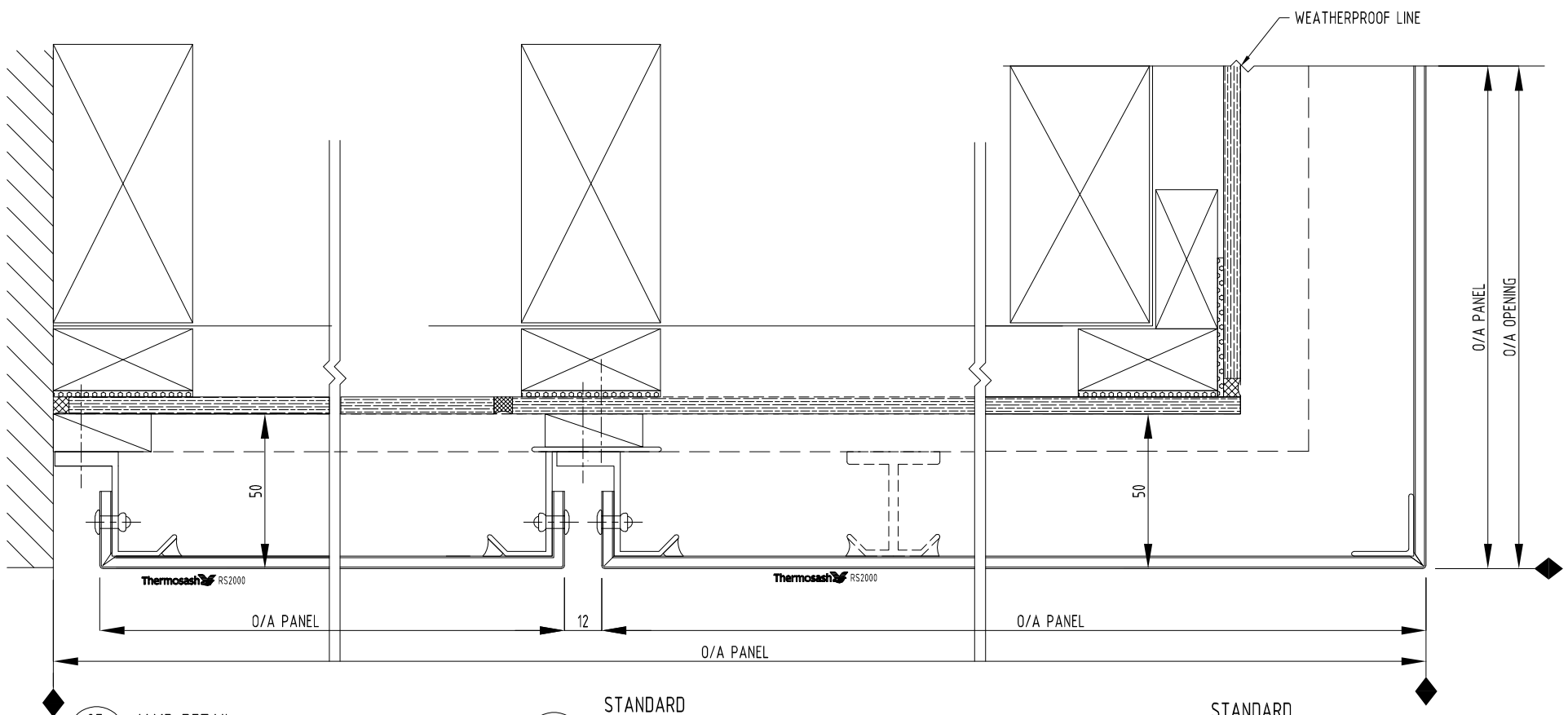
JAMB DETAIL 05/01 1:2
